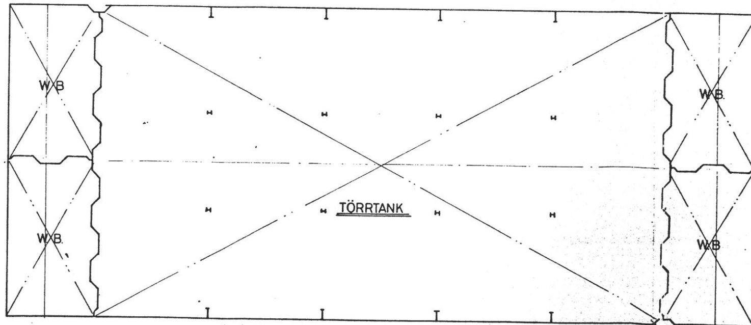
SNITT UNDER LASTEDEKK
